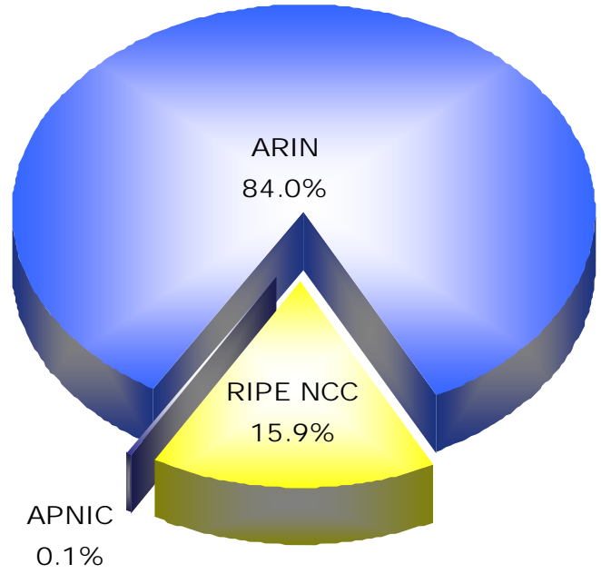
IPv4
